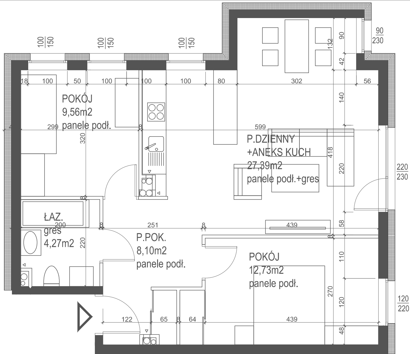
mieszkanie nr 1 pow. 62,05m 2 poziom ±0,00 skala 1:50
